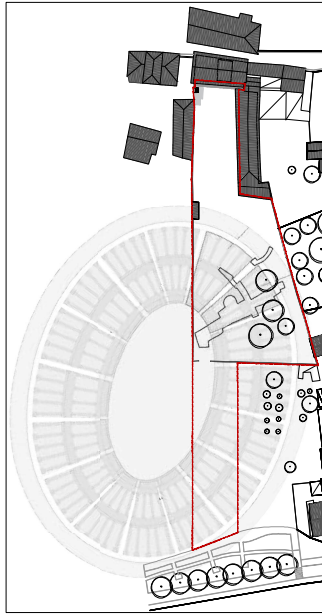
sovraposizione dell'area di progetto con la damieristica ricostruttiva dell'edificio
