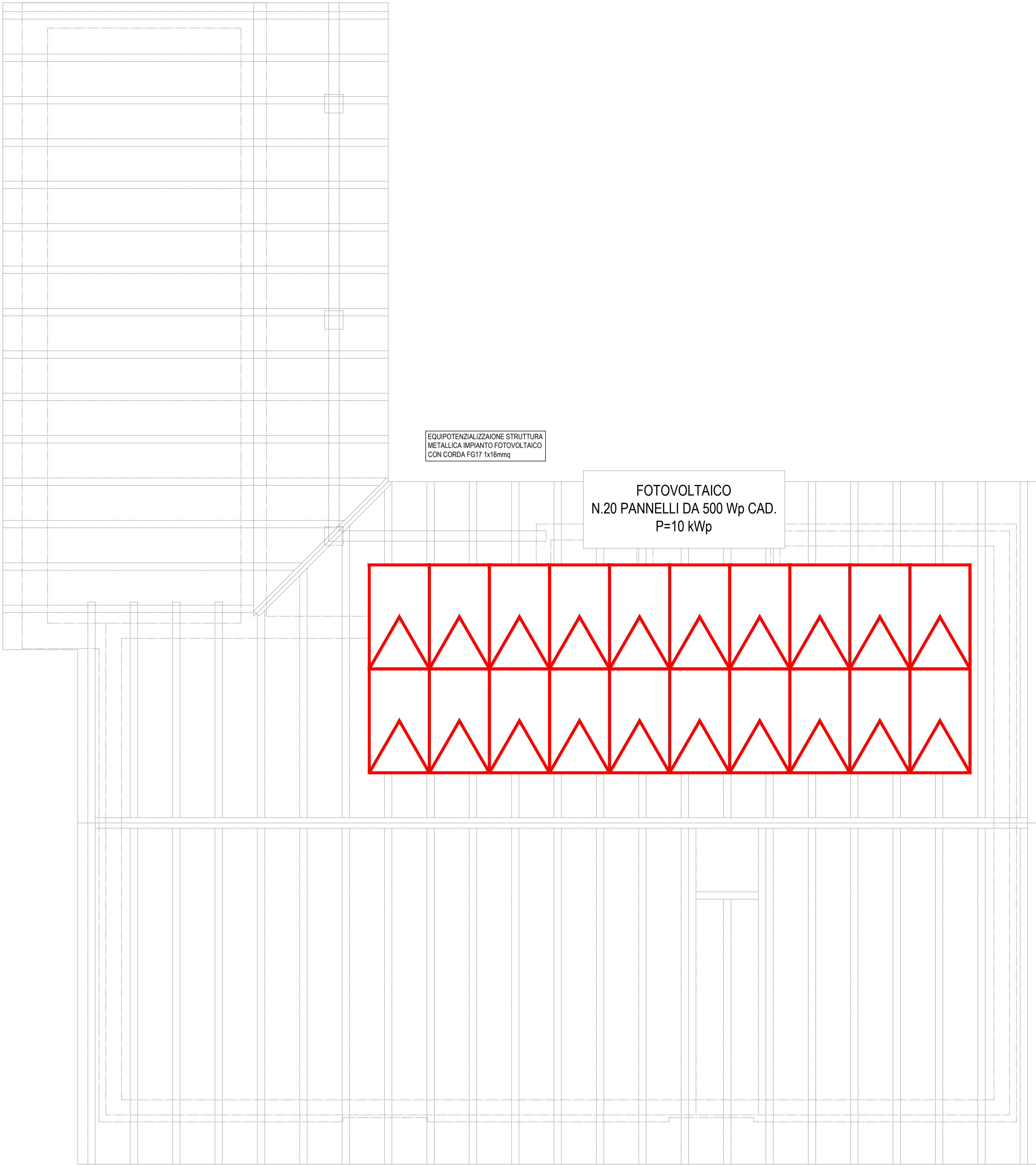
PIANTA COPERTURA SCALA 1:50
