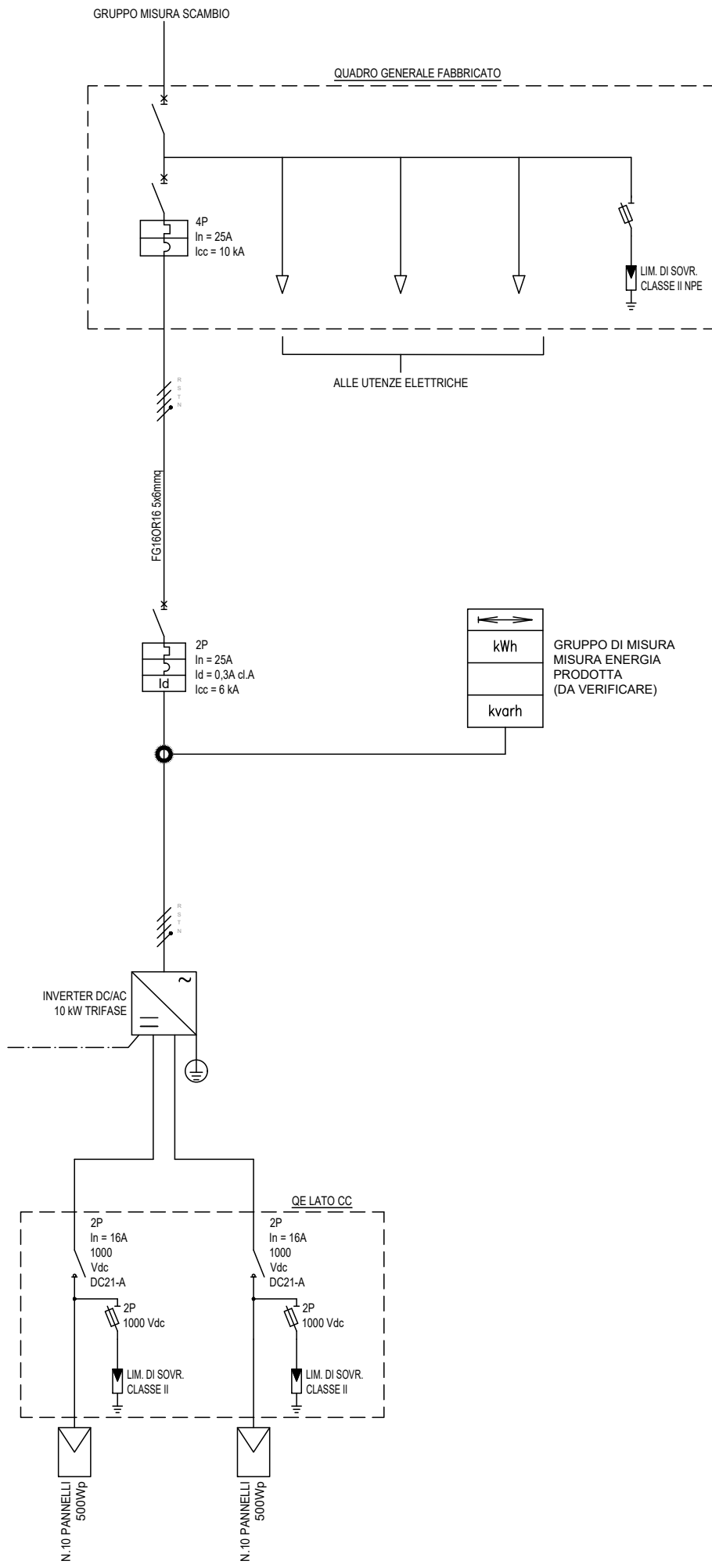
SCHEMA UNIFILARE FOTOVOLTAICO
