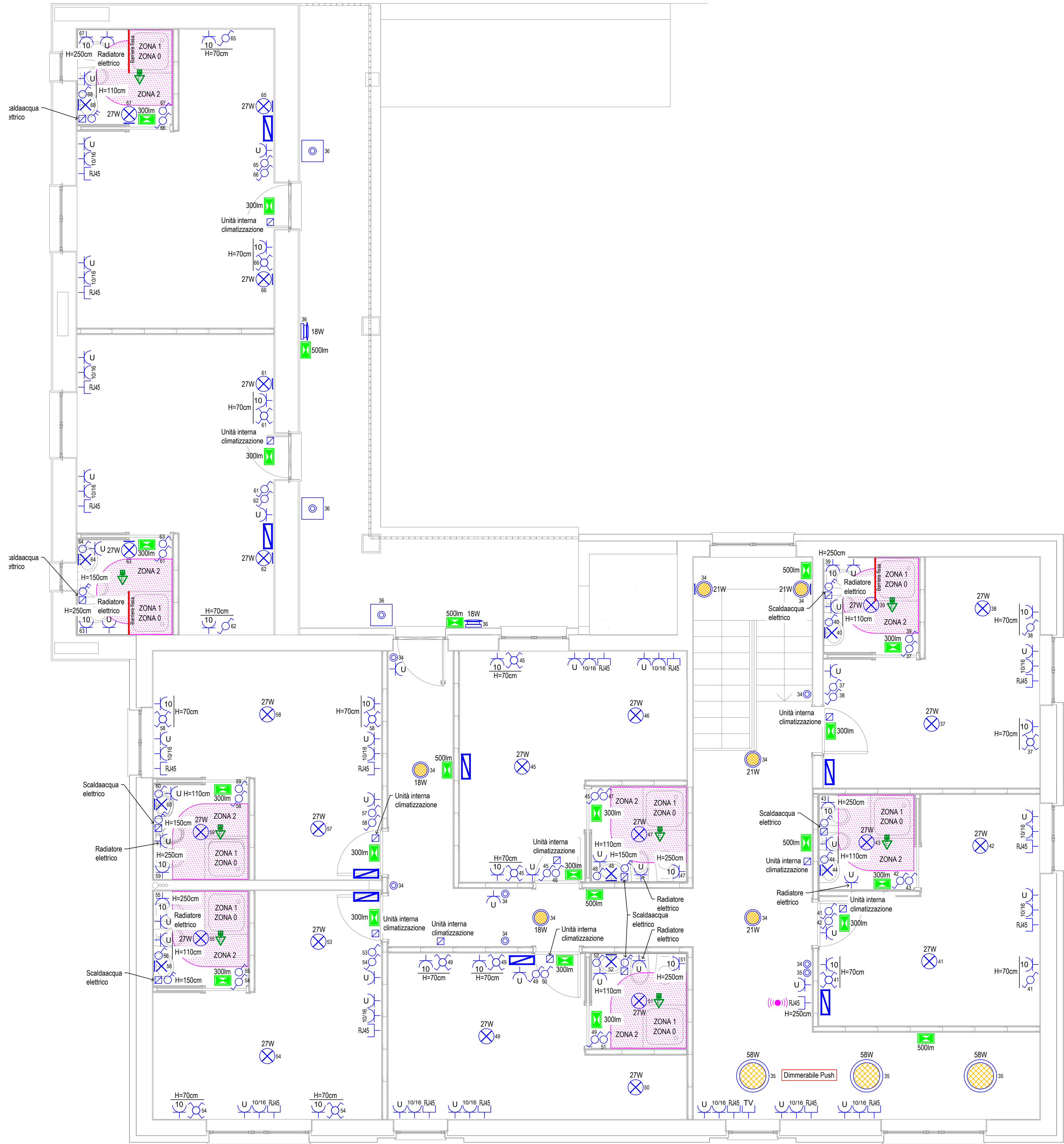
PIANTA PIANO PRIMO SCALA 1:50
