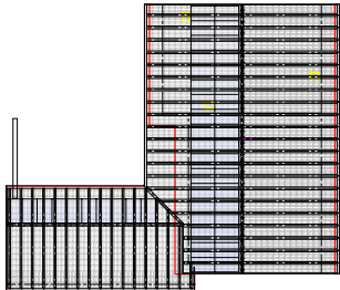
PIANTA COPERTURA 1:200
