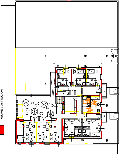
PIANTA PIANO TERRA 1:200
