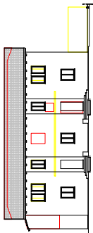
PROSPETTO SUD-OVEST SU VIA PIER SILVERIO LEICHT 1:200
